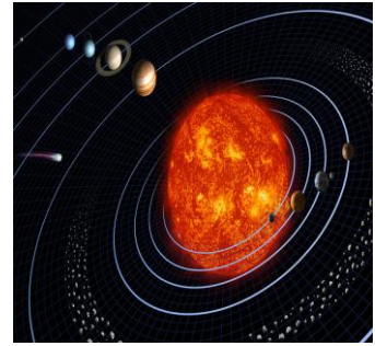
٤- المجموعة الشمسية
